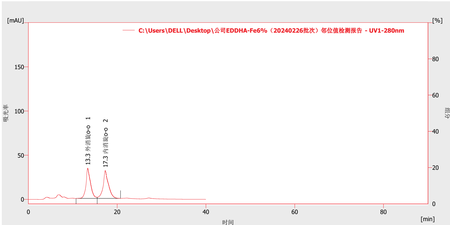
结果表 (ES1D - C:\Users\DELL\Desktop\公司EDDHA-Fe6% (20240226批次) 邻位值检测报告 - UV1-280nm)
