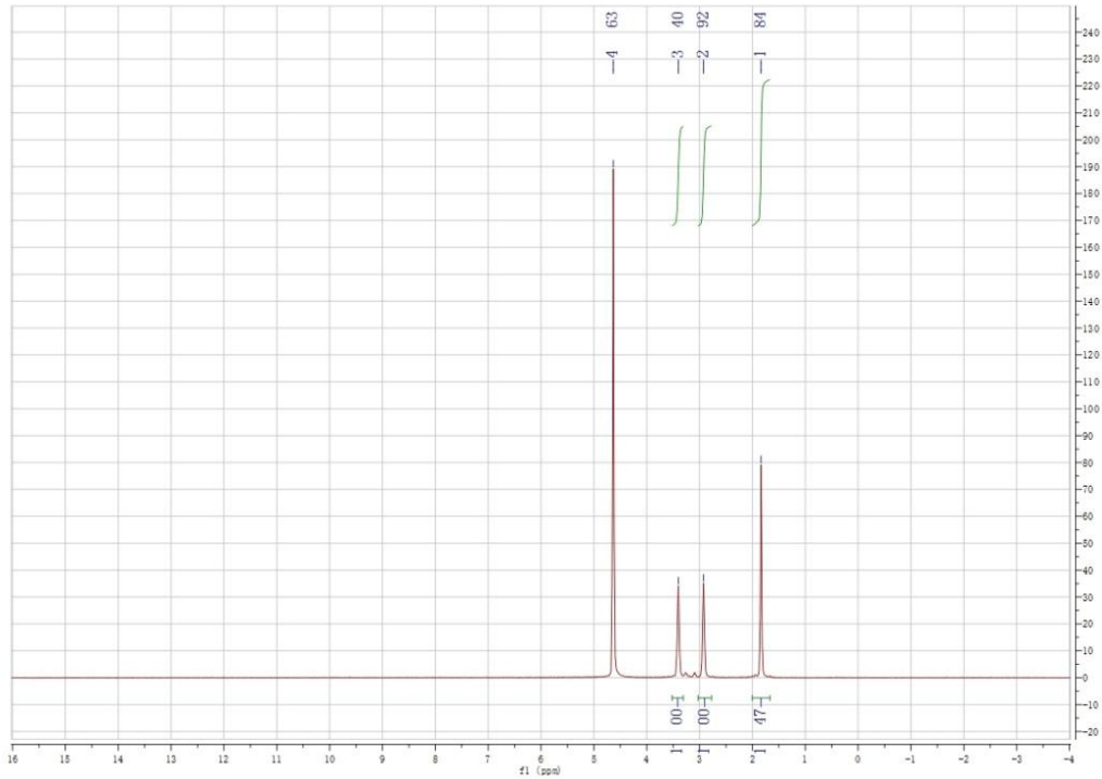
Fig.3 ^1\text{H} NMR spectrum 图 3 乙酰牛磺酸镁核磁共振氢谱图
